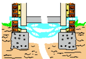
Zavěšené, dobře větrané podloží
