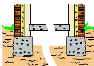
Zavěšené, nevětrané podloží
